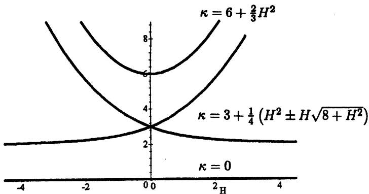
Fig. 1 (H, \kappa)
